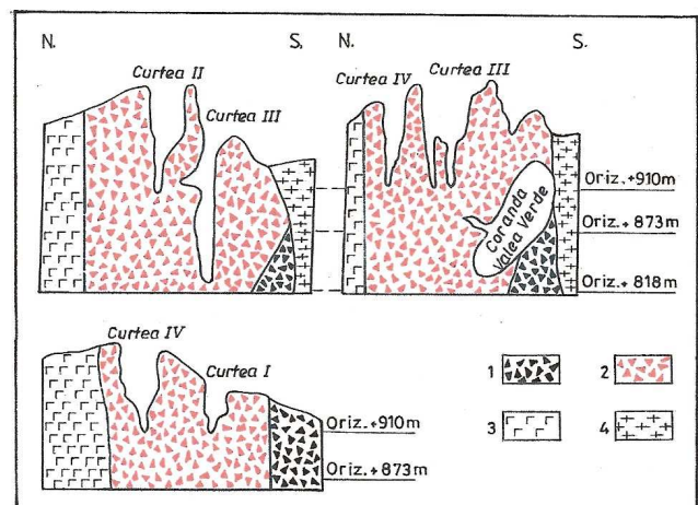
Legendă : 1. Breția neagră ; 2. Breția de Cetate ; 3. Riolite ; 4. Gresii conglomerate Légende : 1. Brèche noire ; 2. Brèche de Cetate ; 3. Ryolithes ; 4. Conglomerats de grès
