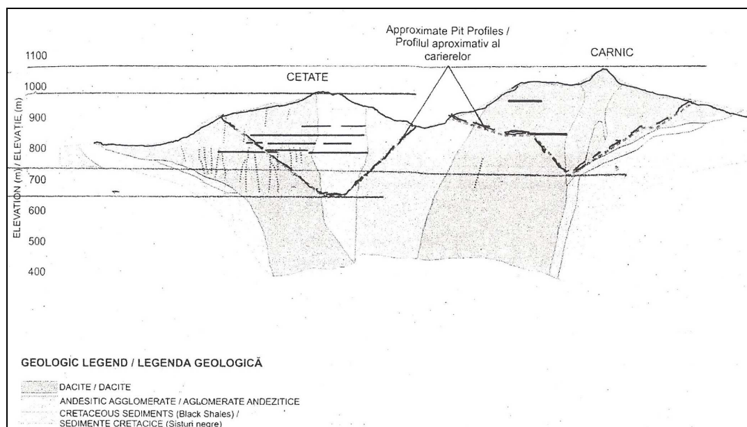
Figura 5. Secțiune geologică schematică prin zonele Cărnic și Cetate de la Roșia Montană. Figure 5. Coupe géologique schématisée des zones de Cărnic et Cetate de Roșia Montană
